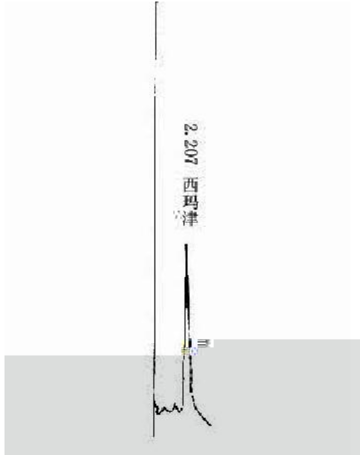
图A1 西玛津标准品色谱图
